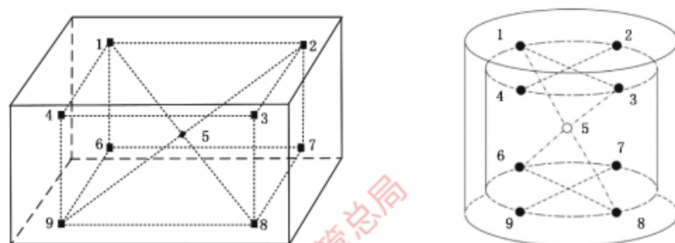
图2 工作空间深度大于15 cm时的温度测量点分布示意图
