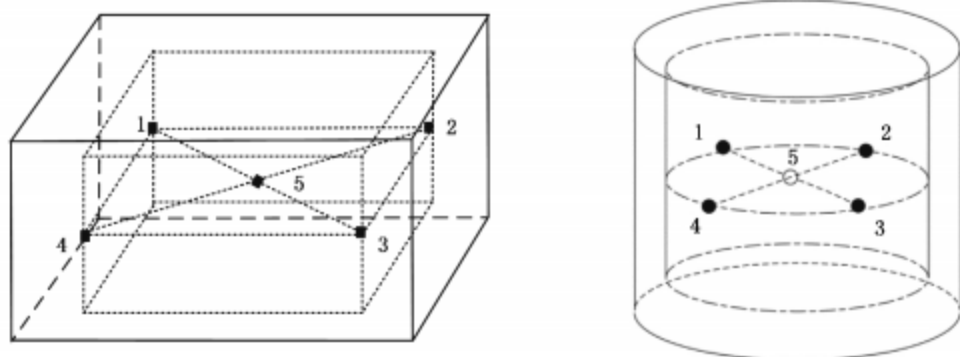
图1 工作空间深度小于15 cm时的温度测量点分布示意图
